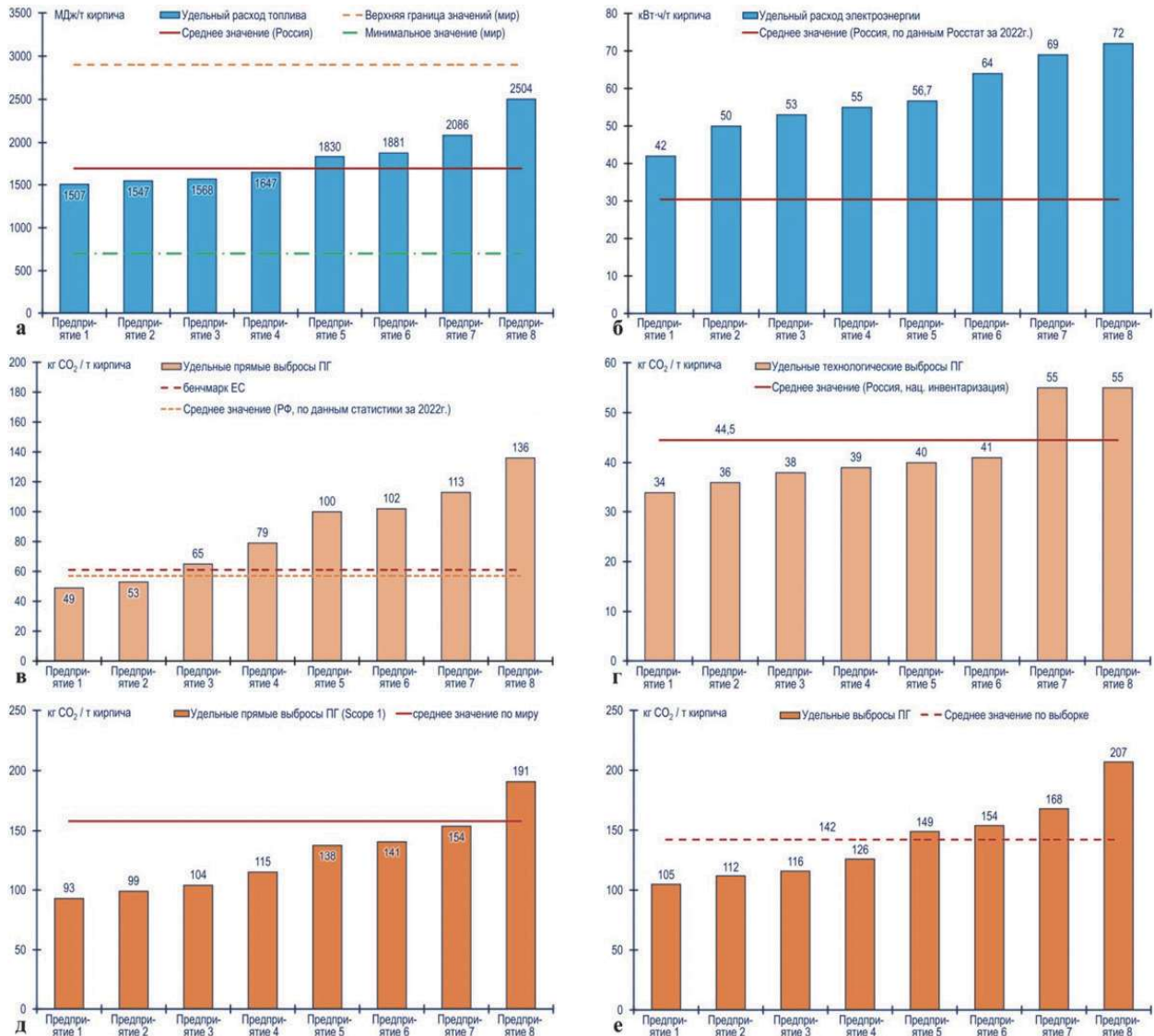
Рис. 4. Кривые бенчмаркинга по удельным расходам энергии и выбросам ПГ при производстве кирпича, построенные с применением системы Бенчмарки РПИЧ нг:
